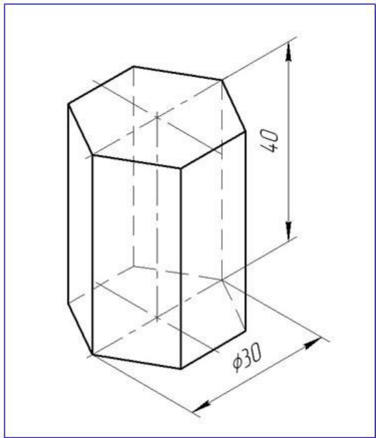
АксонOMETрический чертeж
